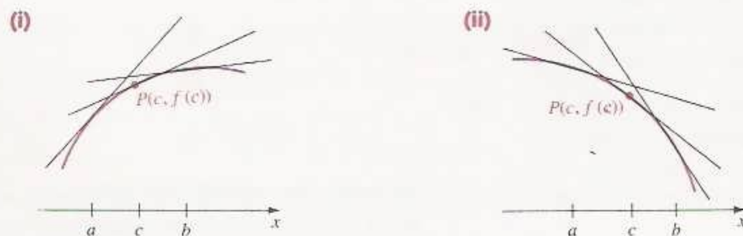
FIGURA 4.24 Concavidad hacia abajo
